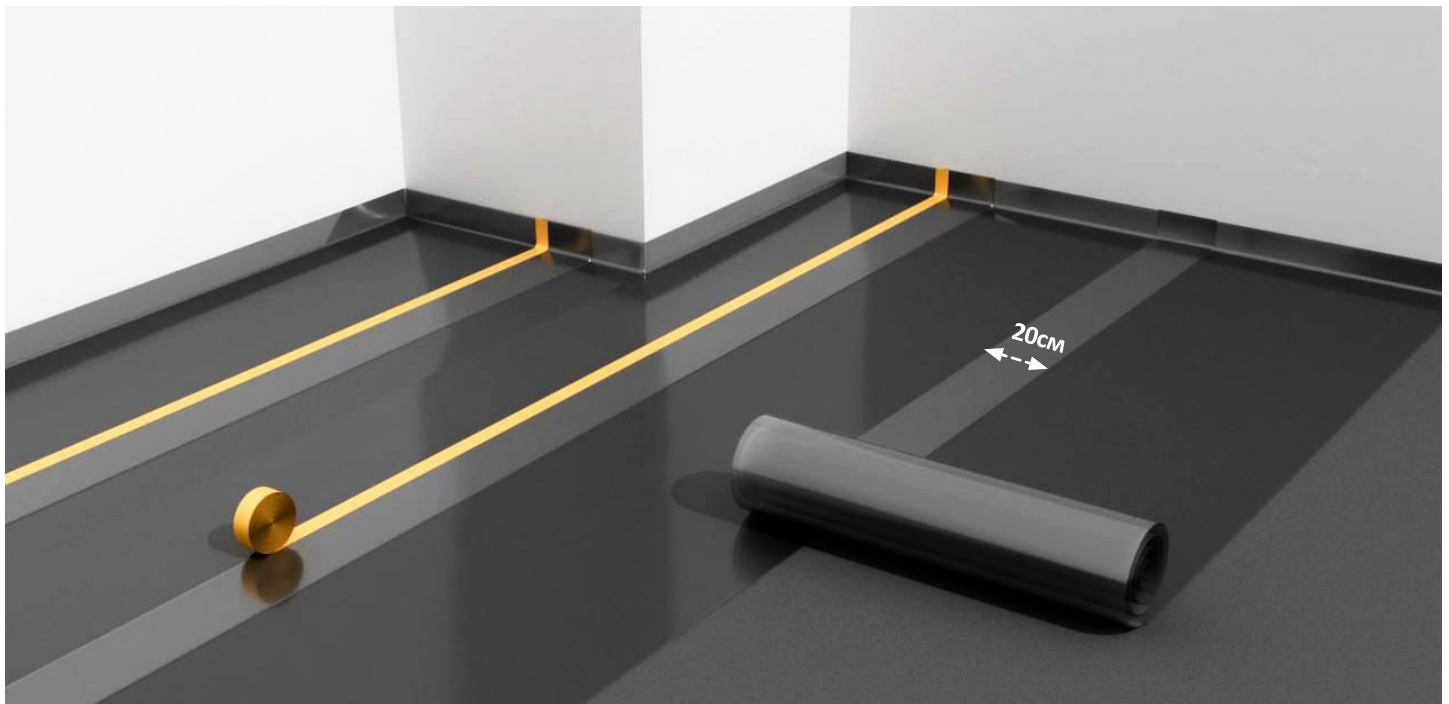
ШАГ 1: установка пароизоляции
